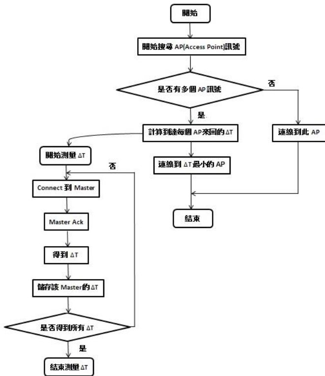
圖五: 程式流程圖
