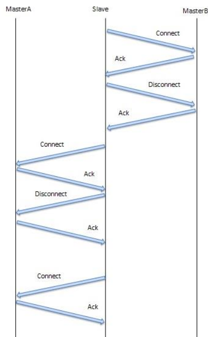
圖四:狀況乙：受困人員端接收到多位救難人員端的訊號(在此以兩位救難人員端為例)
