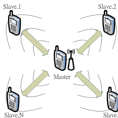
圖一：WiFi-SoftAP 階層式群集(Hierarchical Cluster)架構圖
