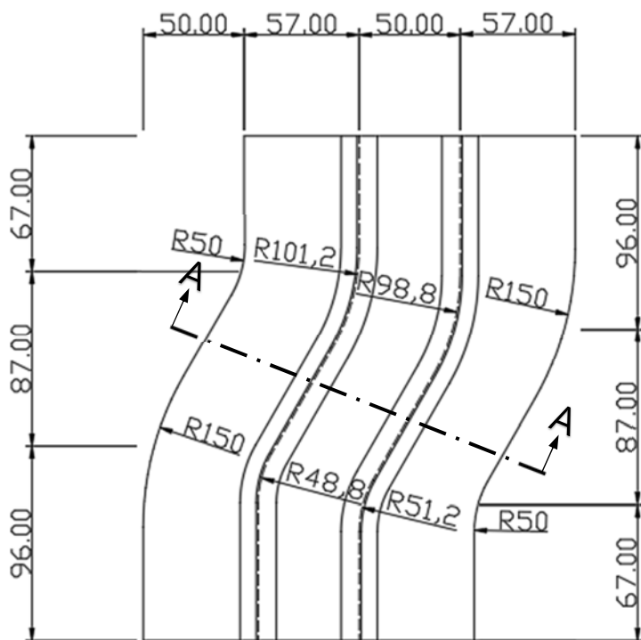
(b)產品尺寸及 A-A 剖面圖
